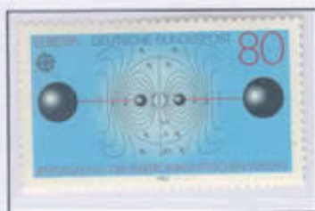
Onde elettromagnetiche
